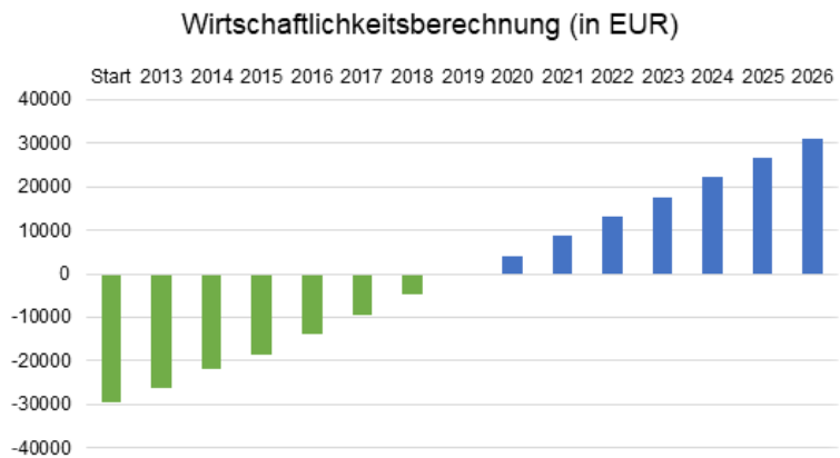
Wirtschaftlichkeitsberechnung für die PV-Anlage Volksschule
